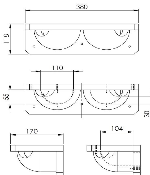
Illustration 2 : dimensions StoElement Fauna SW-F 20
