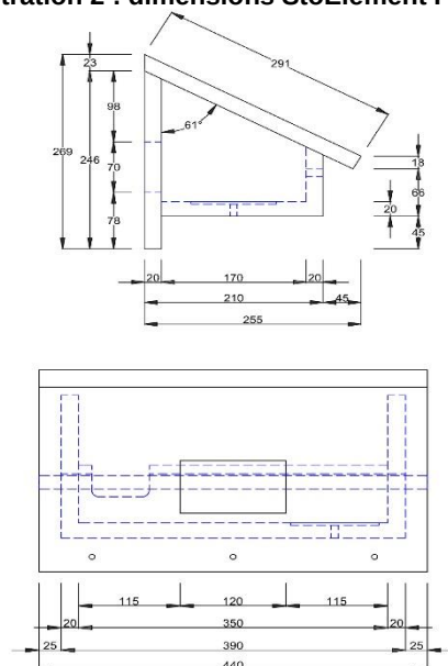
illustration 2 : dimensions StoElement Fauna MS-F 20
