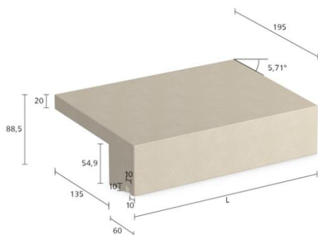
StoDeco Frame F - type AF P.195
