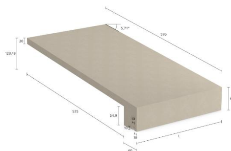
StoDeco Frame F - type AF P.595
