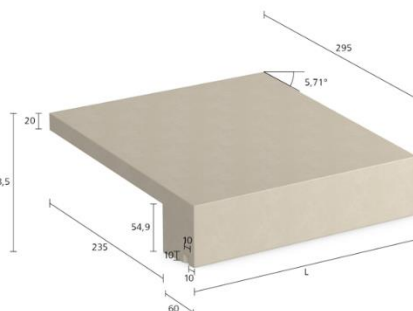
StoDeco Frame F - type AF P.295
