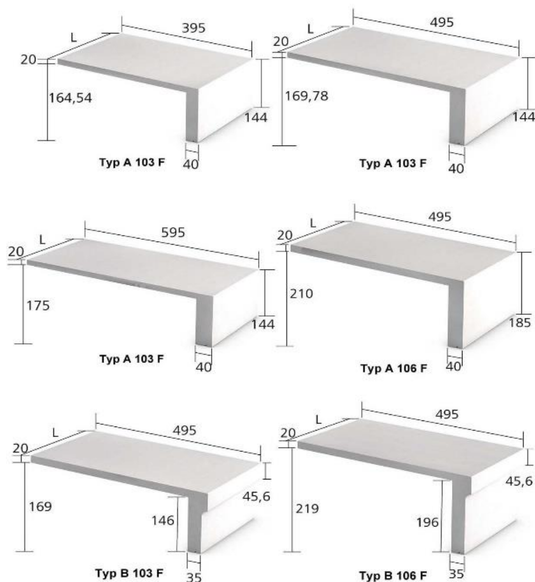
Gamme StoDeco Frame - F Type A/B
