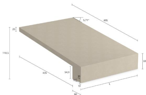
StoDeco Frame F - type AF P.495
