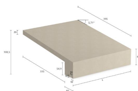
StoDeco Frame F - type AF P.395
