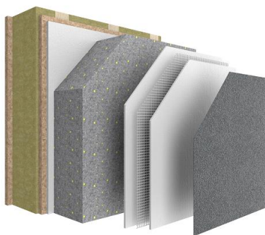
Système StoTherm Classic® sur COB Sous avis technique depuis plus de 10 ans, ce système est devenu une référence sur le marché.
