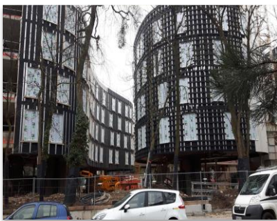
La sous-structure Sto est mise en œuvre en système mixte avec une ossature verticale métallique et une ossature horizontale cintrée en bois.
