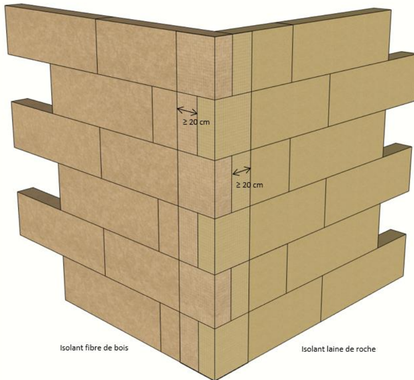
Figure 5 : Jonction entre les systèmes StoTherm Wood 2 bis et StoTherm Vario 1 en angle de bâtiment
