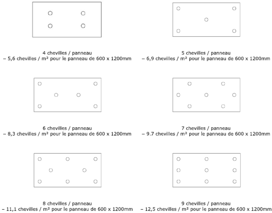
Figure 22 – Exemple de plans de fixation sur CLT (1/2) (espacement entre vis à rosace ≥ 150mm et distance au bord ≥ 150 mm)
