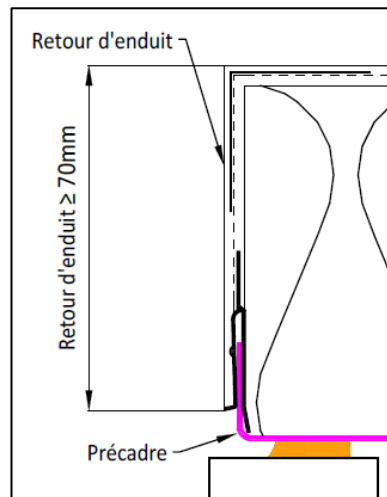
Figure 25 – Aperçu de la cote de retour d'enduit
