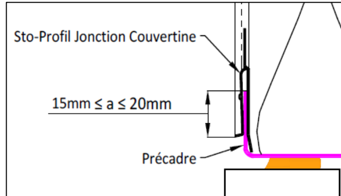
Figure 24 – Aperçu de la cote d'enfoncement du précadre dans le Sto-Profil Jonction Couvertine
