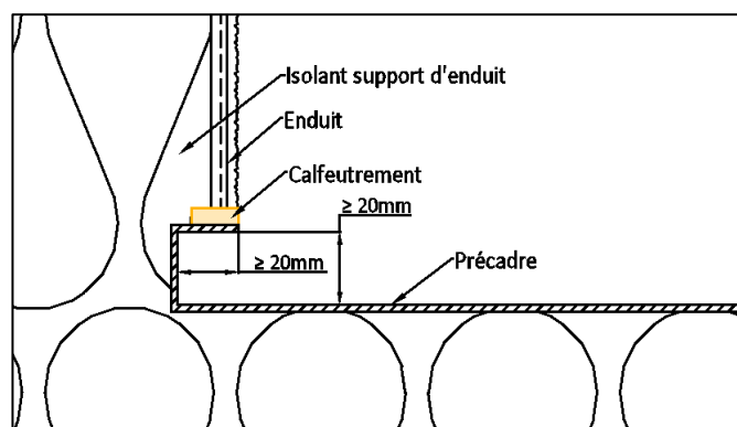
Figure 26 – Principe de réalisation de la partie pièce de capotage
