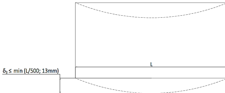
Figure 18 – Représentation du critère de flèche nuisible à respecter pour la structure d'appui en pied de COB »
