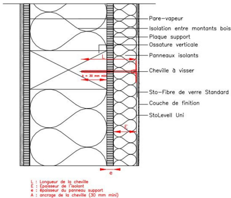
Figure 20 - Fixation des panneaux isolants par vis avec rosace (coupe verticale) dans les montants de l'ossature bois
