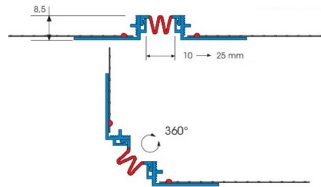
Figure 11 - Profil apu w 56 movi
