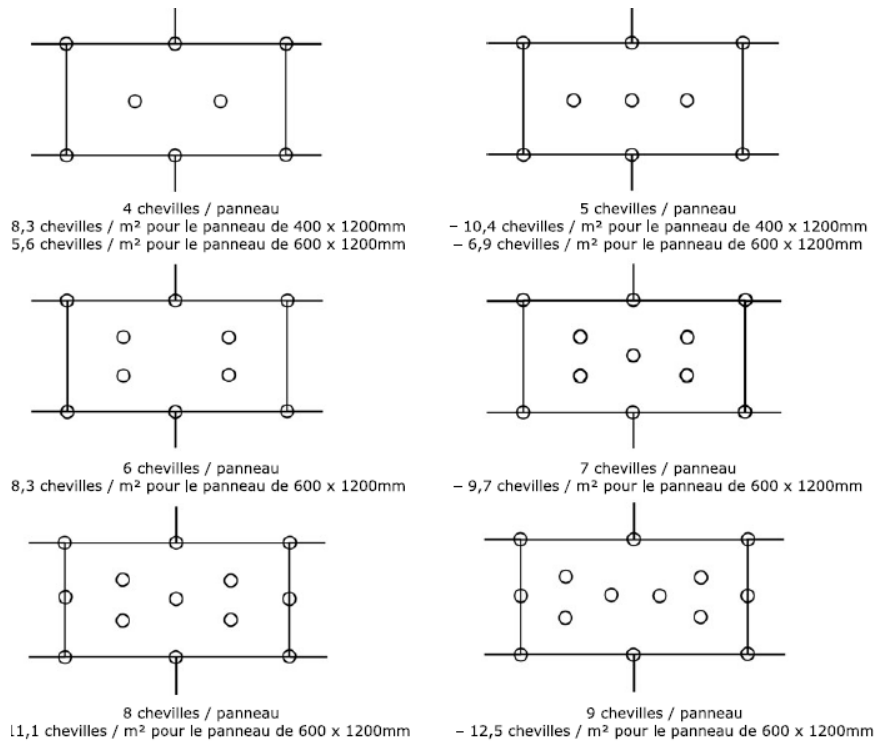
Figure 22 – Exemple de plans de fixation sur CLT (1/2) (espacement entre vis à rosace ≥ 150mm et distance au bord ≥ 150 mm)
