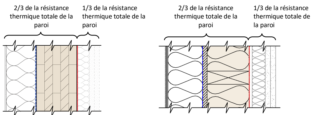
Figure 15 - Schéma de principe de la règle dite des « 2/3-1/3 »
