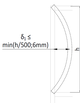
Figure 16 - Représentation du déplacement limite hors plan
