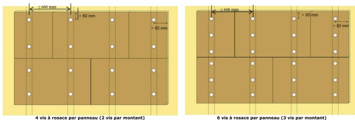
Figure 21 – Plan de fixation pour support COB en partie courante
