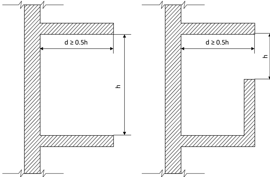
Figure 29 - Définition des éléments architecturaux de protection
