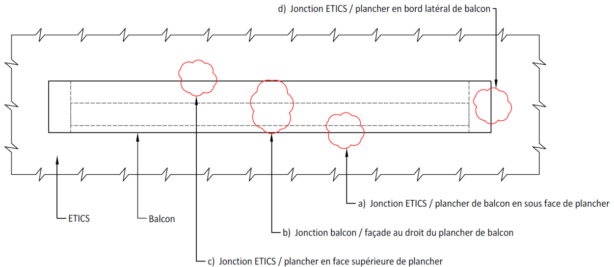
Figure 27 – Aperçu des jonctions ETICS / balcon ou coursive sur une élévation
