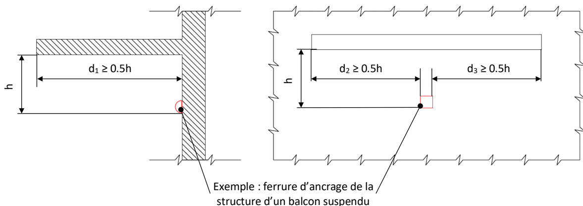
Figure 28 - Représentation des critères de protection des traversées ponctuelles de l'ETICS par une ferrure d'assemblage ou poutre
