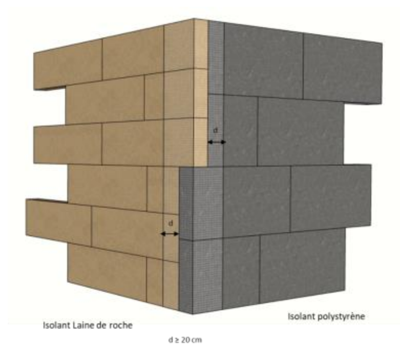
Figure 16a : Système StoTherm Brick LDR avec panneaux en laine de roche de dimensions 600 x 1200 mm
