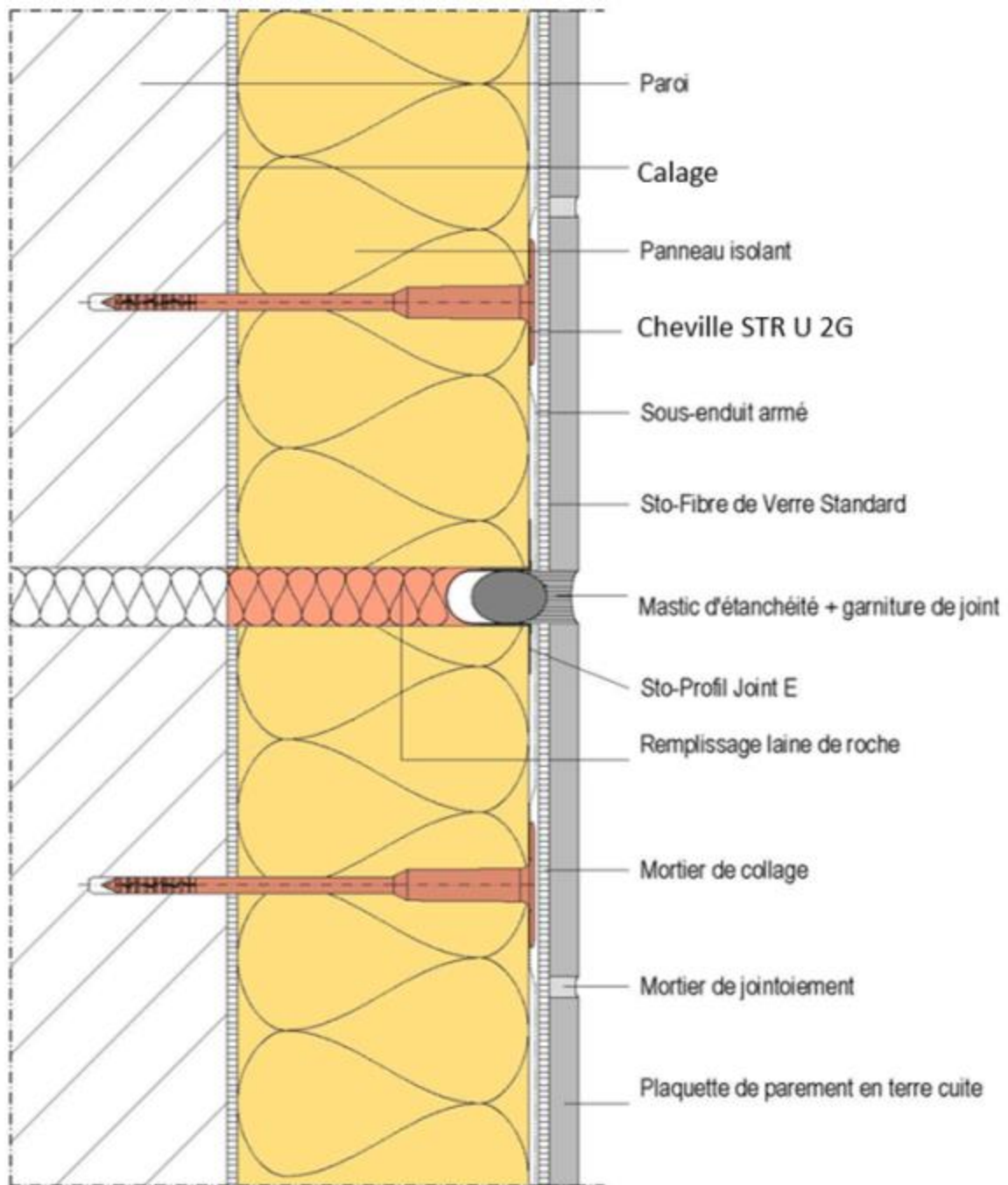
Figure 7b : Utilisation de Sto-Profil Joint type E et mastic d'étanchéité
