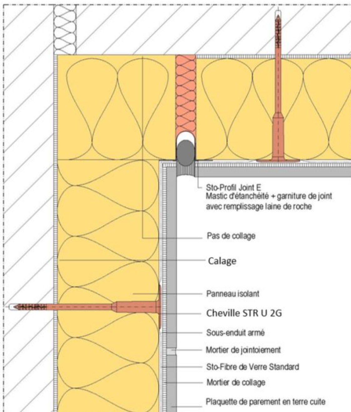
Figure 7c : Utilisation de Sto-Profils Joint type E et mastic d'étanchéité (angle)
