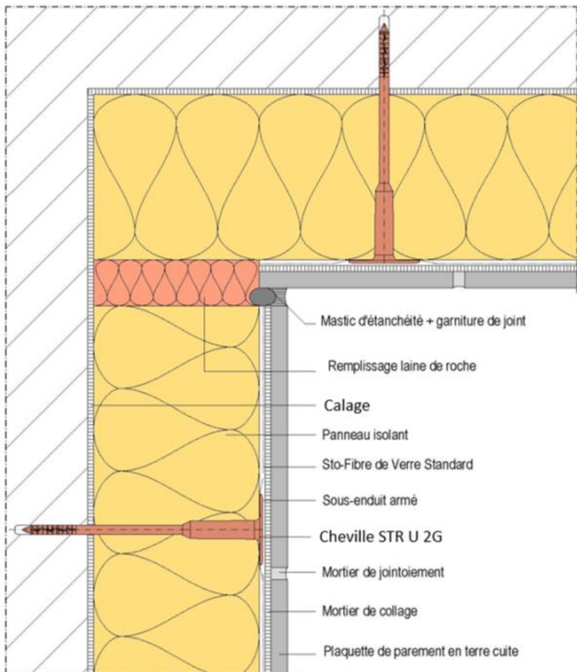
Figure 12 : Traitement des angles rentrants
