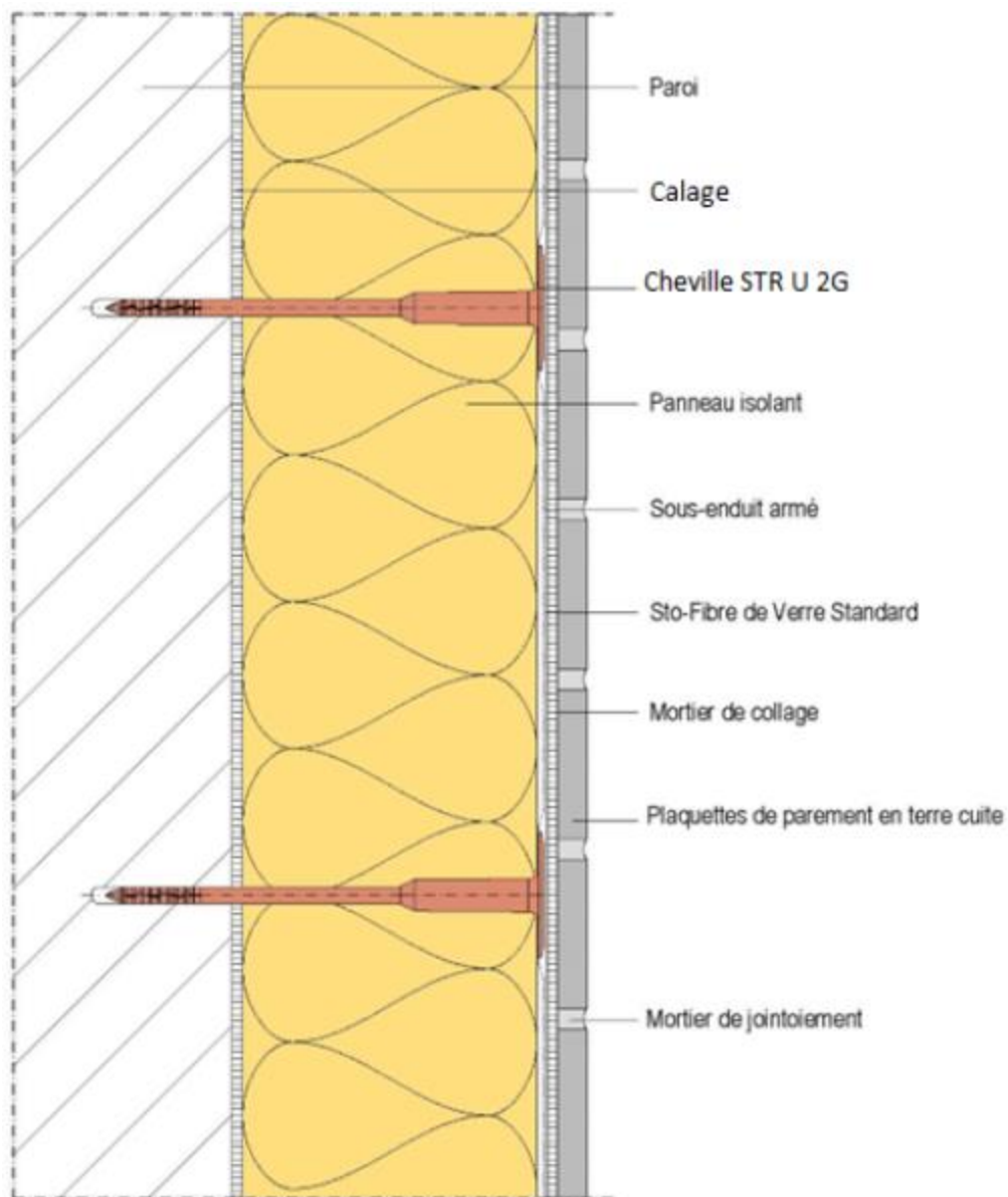
Figure 2 : Principe du système StoTherm Brick LDR
