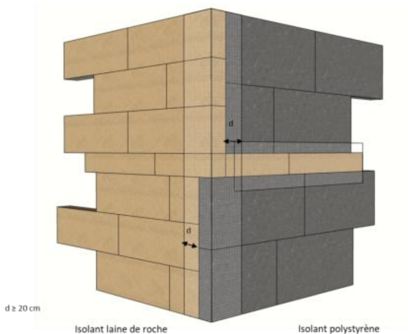
Figure 18a : Système StoTherm Brick LDR avec panneaux en laine de roche de dimensions 600 x 1200 mm
