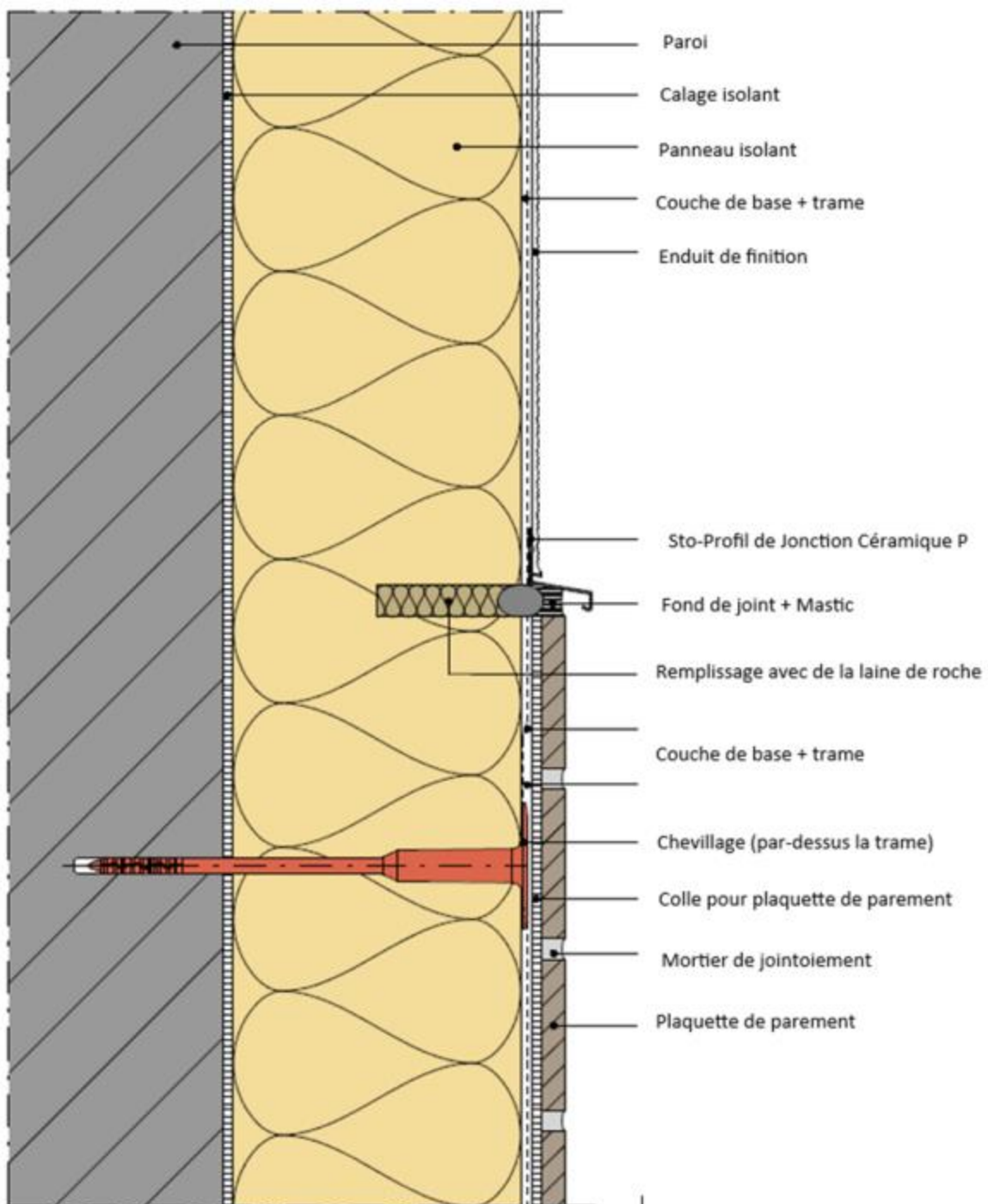
Figure 13a : Finition par plaquettes en partie inférieure
