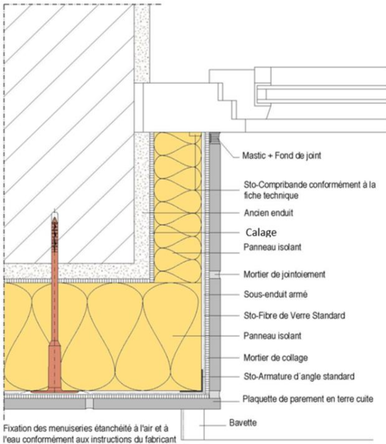
Figure 9c : Raccordement à un élément de menuiserie
