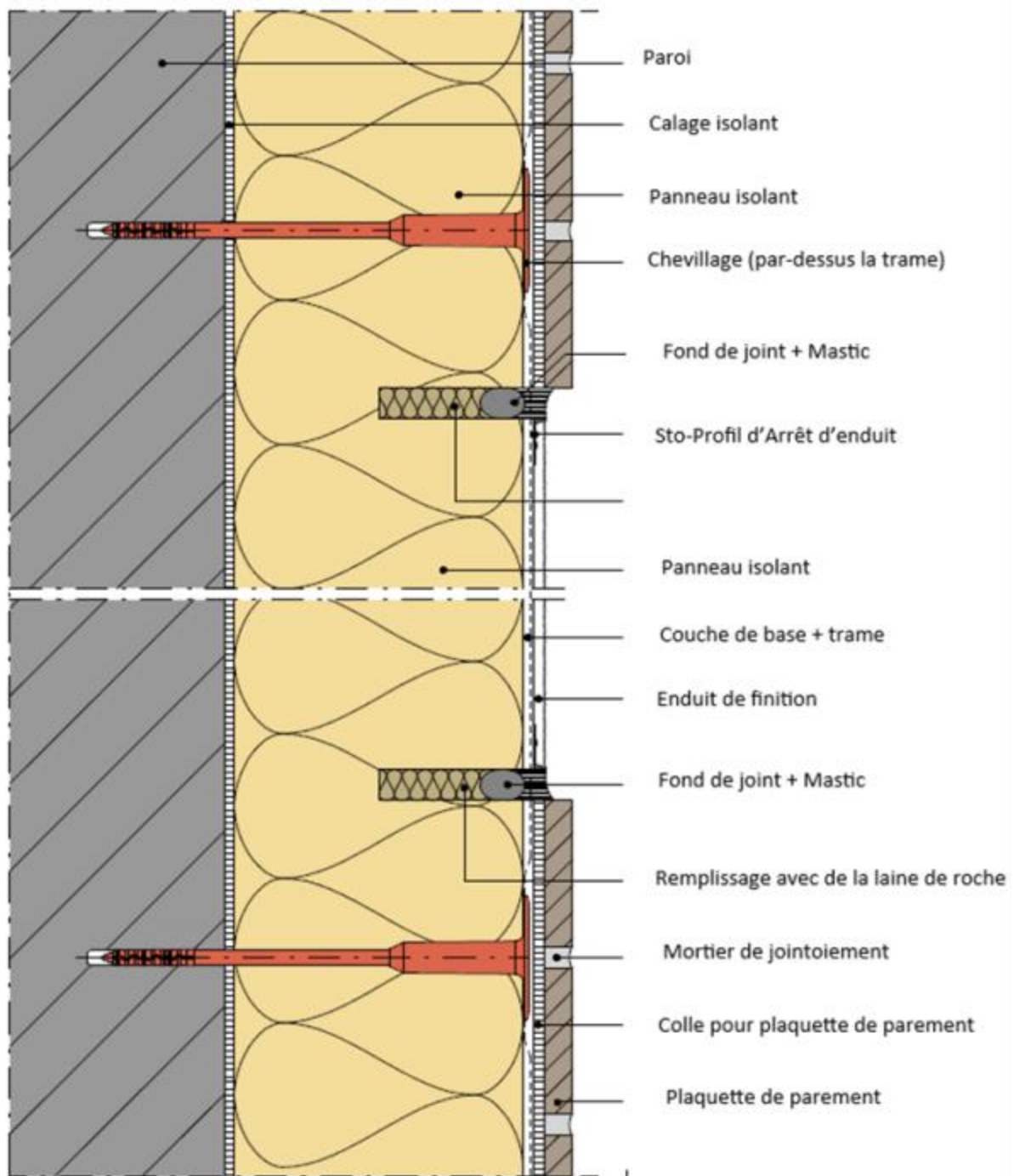
Figure 13b : Raccordement entre finition par plaquette en terre cuite et finition par enduit – isolant continu
