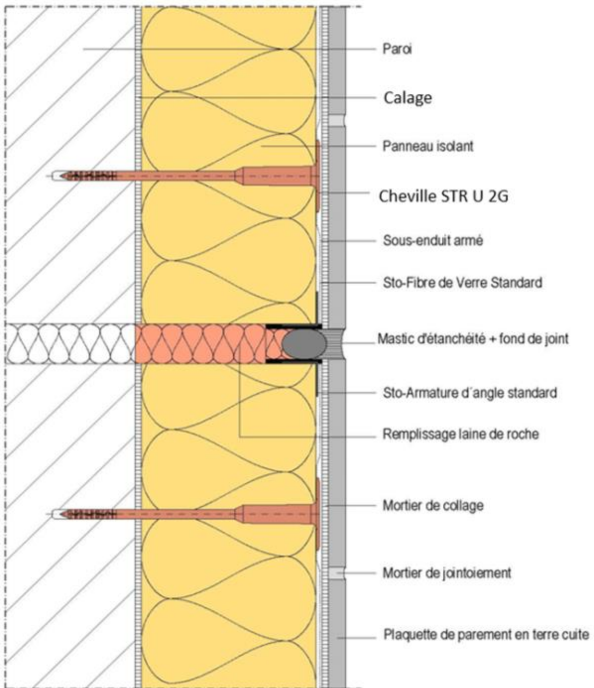
Figure 8 : Traitement du joint de dilatation – Sto-Armature d'angle
