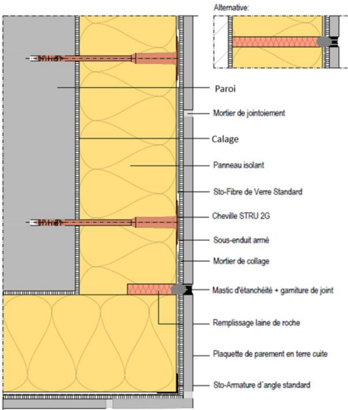
Figure 11 : Traitement des angles sortants
