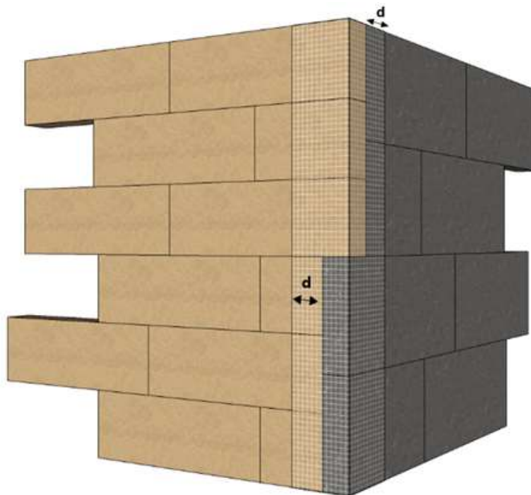
A. Jonction entre des panneaux en PSE et panneaux en laine de roche de dimensions 1200 x 600 mm, en angle de bâtiment
