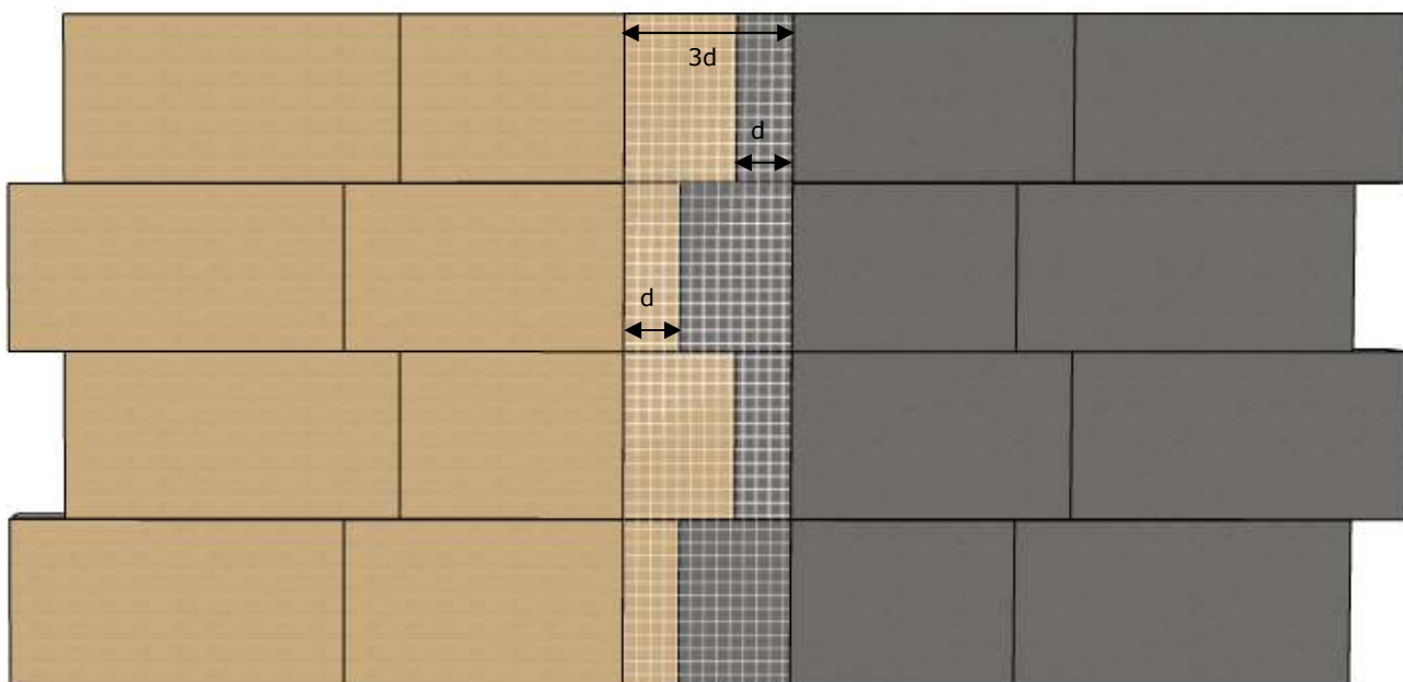
A. Jonction entre panneaux en PSE et panneaux en laine de roche de dimensions 1200 x 600 mm
