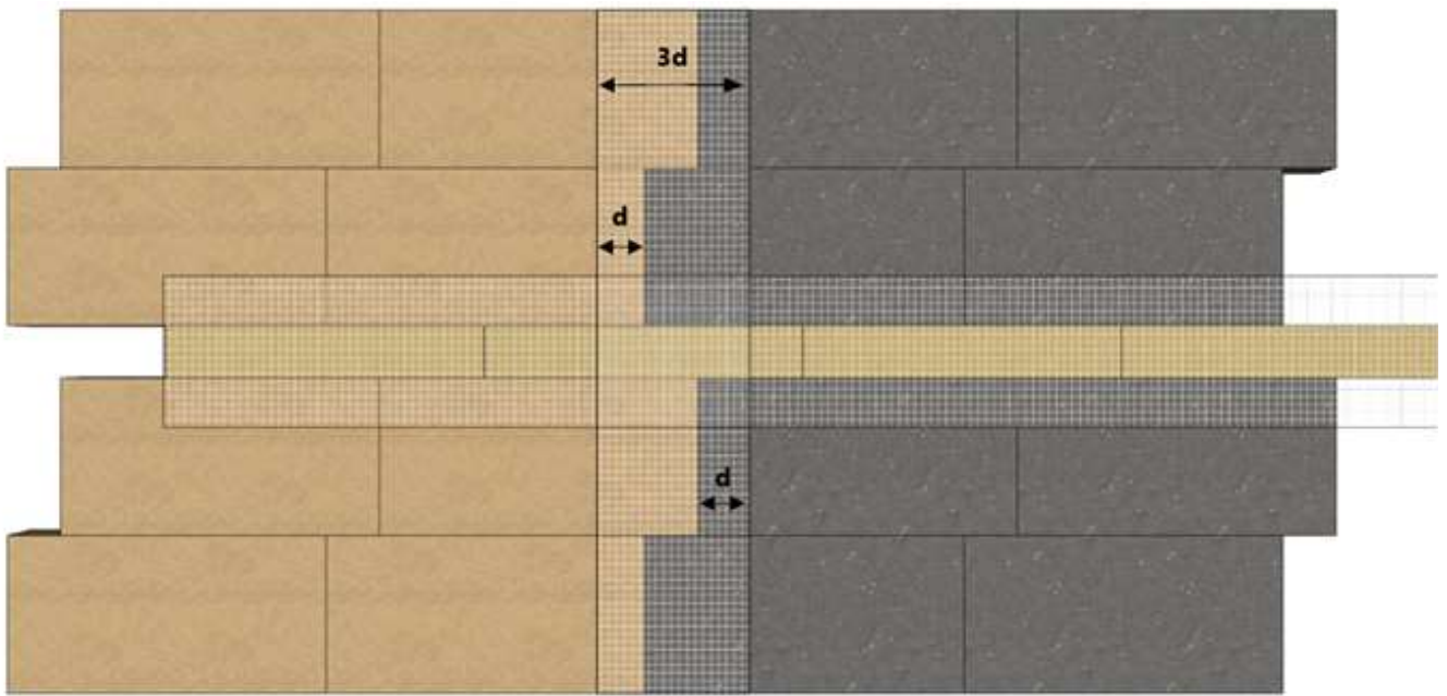
A. Jonction entre des panneaux en PSE et panneaux en laine de roche de dimensions 1200 x 600 mm, avec bande coupe-feu d \geq 200 mm
