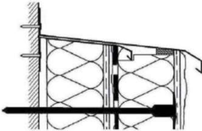
Figure 4a : nouvelle couvertine inversée sans dépose de l'existant
