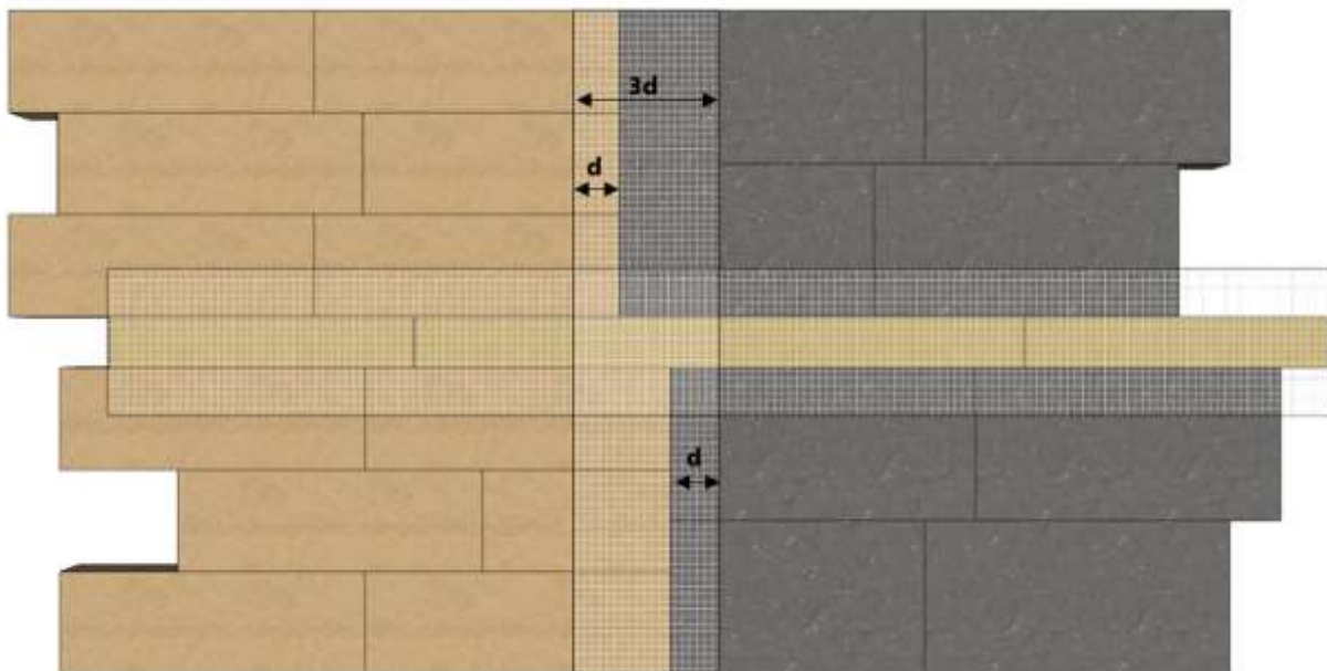
B. Jonction entre des panneaux en PSE et panneaux en laine de roche de dimensions 1200 x 400 mm avec bande coupe-feu d \geq 200 mm
