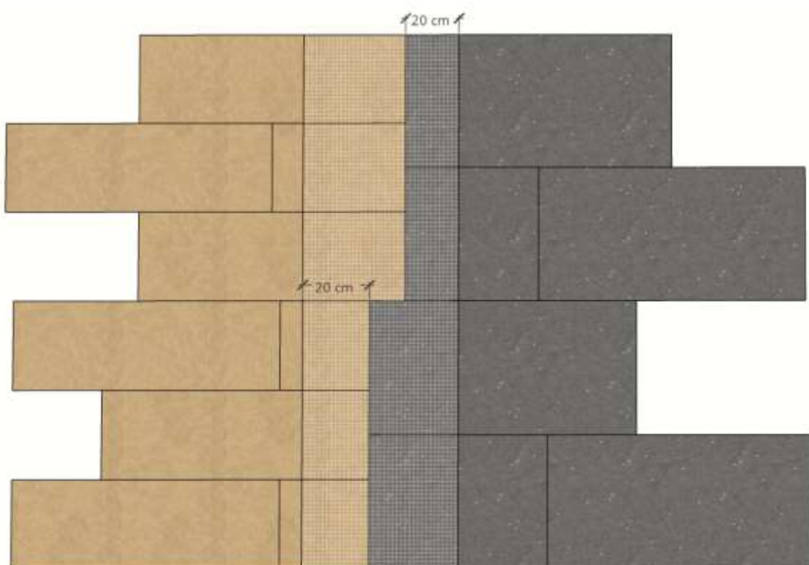
B. Jonction entre panneaux en PSE et panneaux en laine de roche de dimensions 1200 x 400 mm de nature différente
