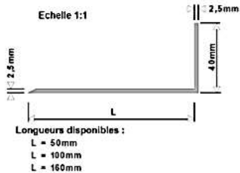
Figure 5a : Profilé de départ en PVC – élément fixé au support : Sto-Profil Départ PH - K
