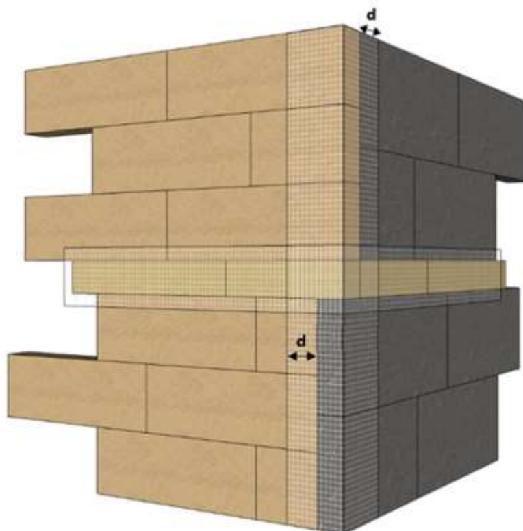
B. Jonction entre des panneaux en PSE et des panneaux en laine de roche de dimensions 1200 x 400 mm avec bande coupe-feu, en angle de bâtiment
