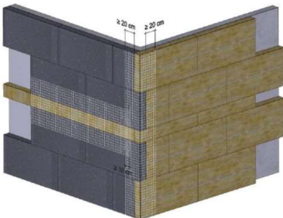
A. Jonction entre des panneaux en PSE et des panneaux en laine de roche de dimensions 1200 x 600 mm avec bande coupe-feu, en angle de bâtiment
