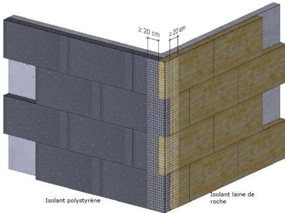
A. Jonction entre des panneaux en PSE et panneaux en laine de roche de dimensions 1200 x 600 mm, en angle de bâtiment
